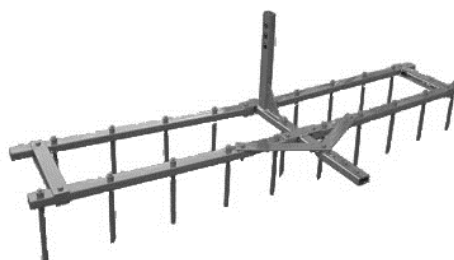
Рисунок А 4 – Борона БР1-2
